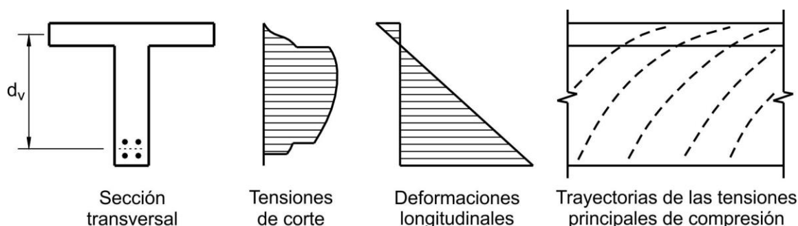
Figura C 5.8.3.4.2-1. Análisis seccional detallado para determinar la resistencia al corte de acuerdo con el artículo 5.8.3.1.
