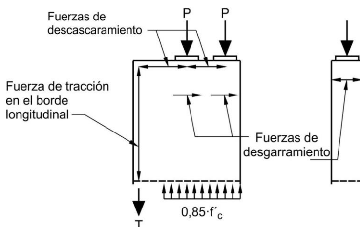
Figura C 5.10.9.3.2-3. Fuerzas de tracción en los bordes
