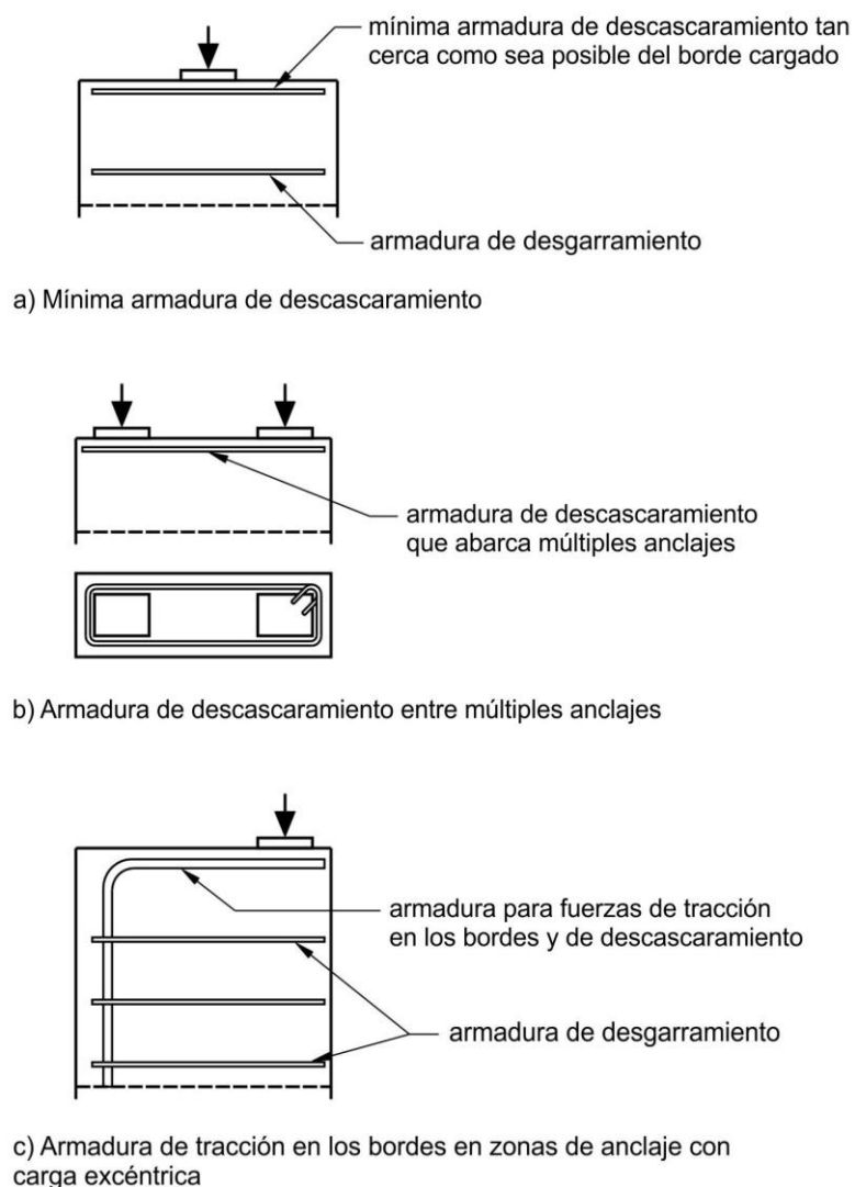
Figura C 5.10.9.3.2-4. Disposición de la armadura en las zonas de anclaje
