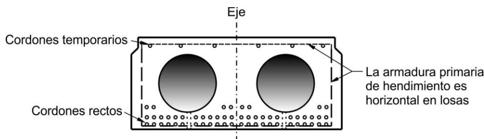
Figura C 5.10.10.1-2. Losa hueca prefabricada
