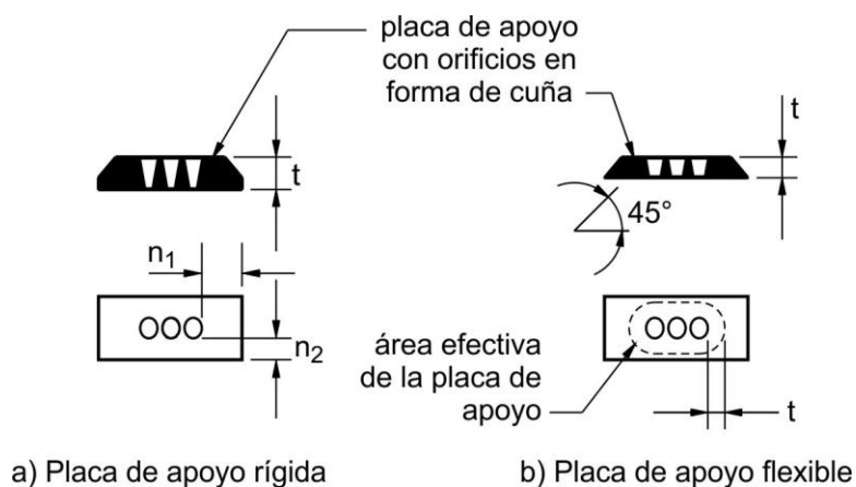
Figura C 5.10.9.7.2-3. Área efectiva de la placa de apoyo para dispositivos de anclaje sin placa de acúñamiento separada
