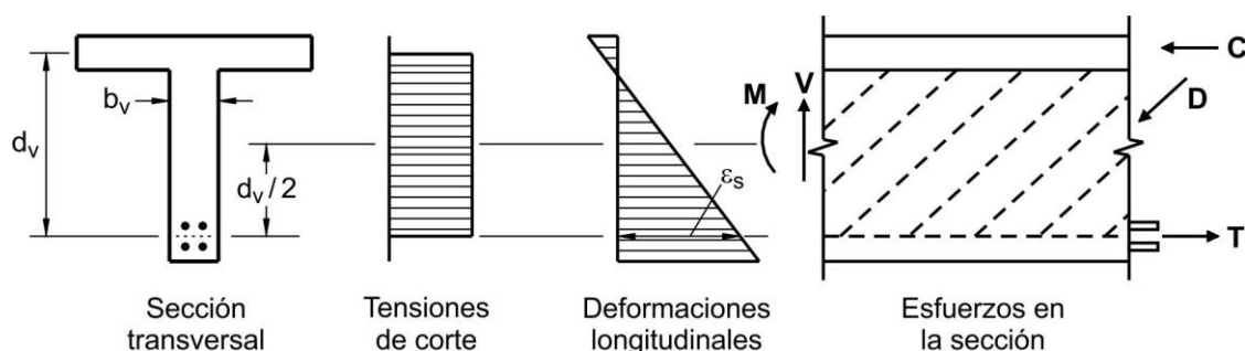
Figura C 5.8.3.4.2-2. Procedimiento más directo para determinar la resistencia al corte de acuerdo con el artículo 5.8.3.4.2
