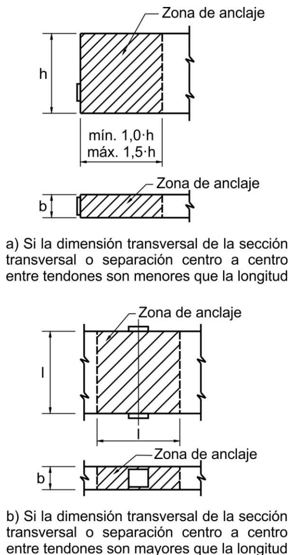
Figura C 5.10.9.1-1. Geometría de las zonas de anclaje
