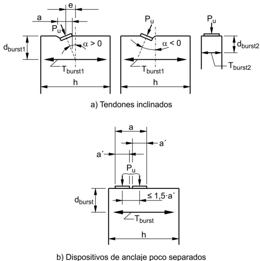
Figura C 5.10.9.6.3-1. Simbología utilizada en las expresiones 5.10.9.6.3-1 y 5.10.9.6.3-2
