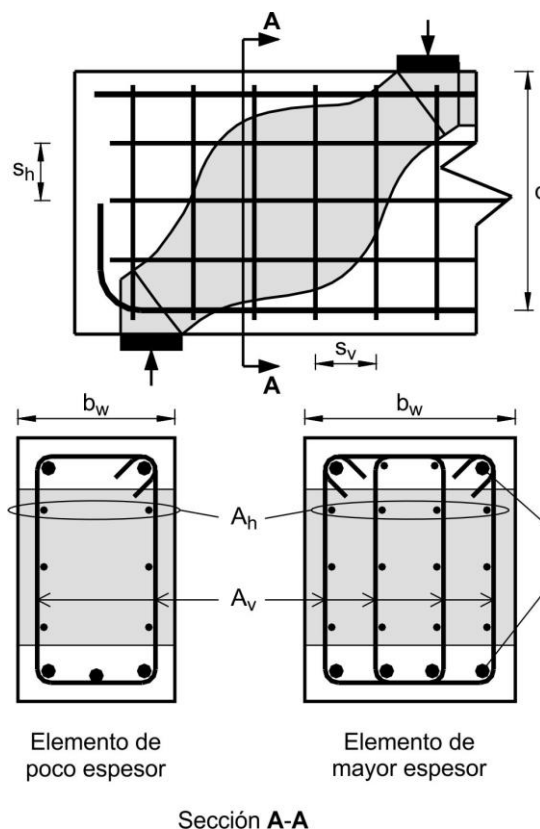
Figura C 5.6.3.6-1. Distribución de la armadura para limitar la fisuración en una biela comprimida
