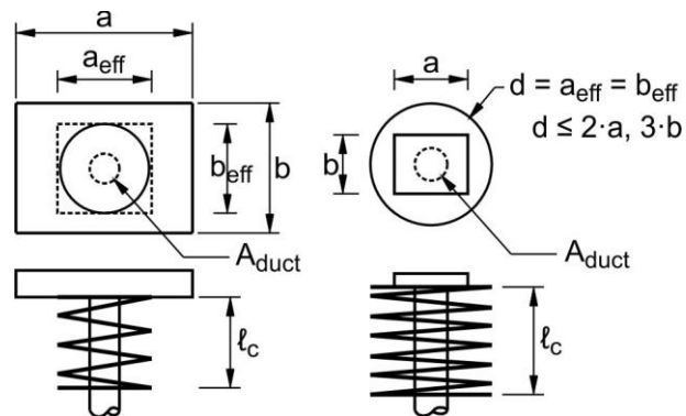
Figura C 5.10.9.6.2-3. Área de apoyo efectiva
