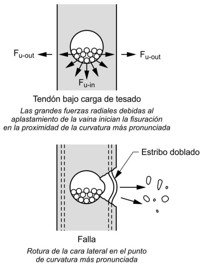
Figura C 5.10.4.3.2-1. Efectos de las fuerzas fuera del plano
