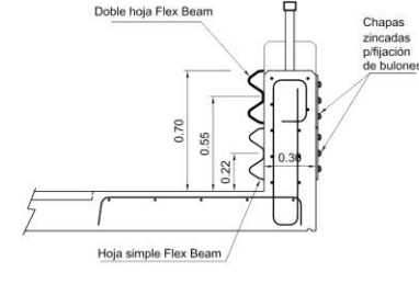
CORTE 5-5 ESCALA 1:20
