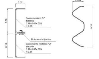
CORTE DEFENSA METÁLICA
