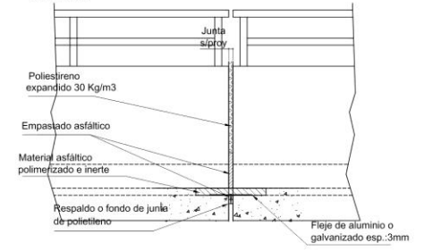
DETALLE JUNTAS ESCALA 1:20
