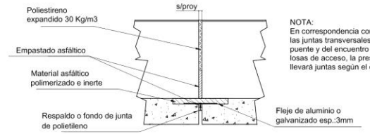
DETALLE JUNTAS ESCALA 1:20
