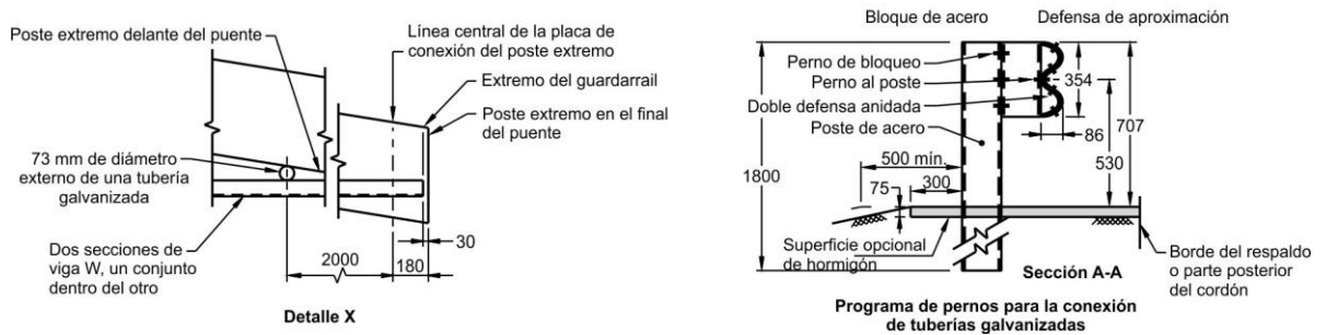
Diseño de defensa protectora en aproximación al puente
