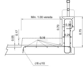
CORTE 4-4 ESCALA 1:20
