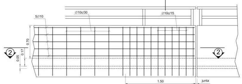
CORTE 2-2 ESCALA 1:20
