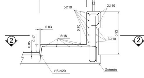
CORTE 3-3 ESCALA 1:20
