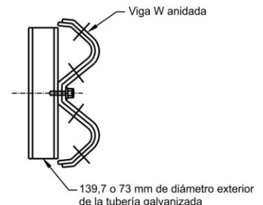
Conexión de la tubería galvanizada
