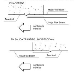
DETALLE DE EMPALME EN ZONA TERMINAL
