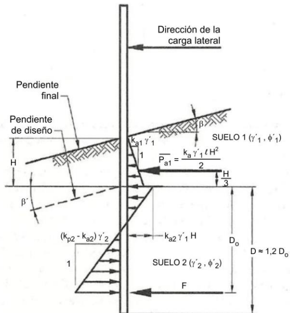
Figura 3.11.5.10-4. Distribución simplificada de empuje de suelo no mayorado para elementos verticales continuos empotrados en suelo granular modificada según Teng (1962).
