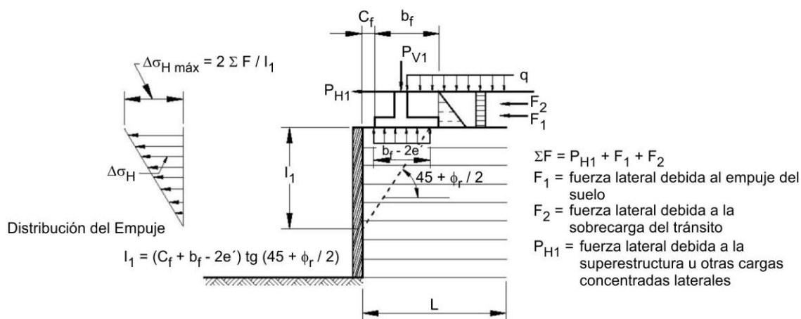
a. Distribución del empuje para el cálculo de la estabilidad interna
