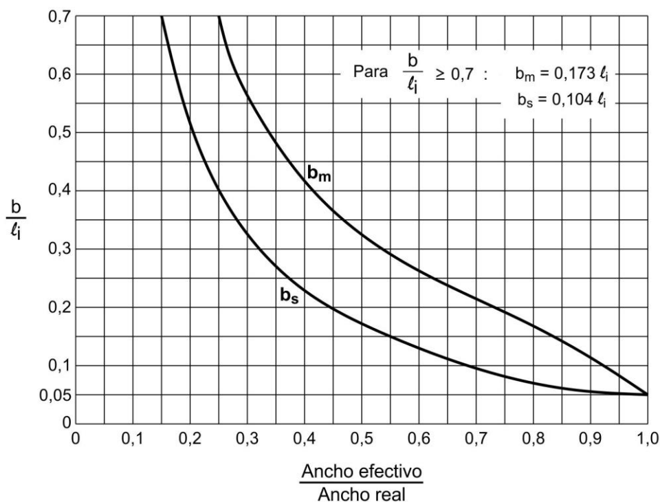
Figura 4.6.2.6.2-2. Valores de los coeficientes del ancho efectivo del ala para el cálculo de b_m y b_s , dado los valores indicados de b/\ell_i .
