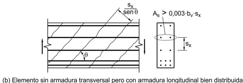
Figura 5.8.3.4.2-3. Definición del parámetro de separación de las fisuras, s_x
