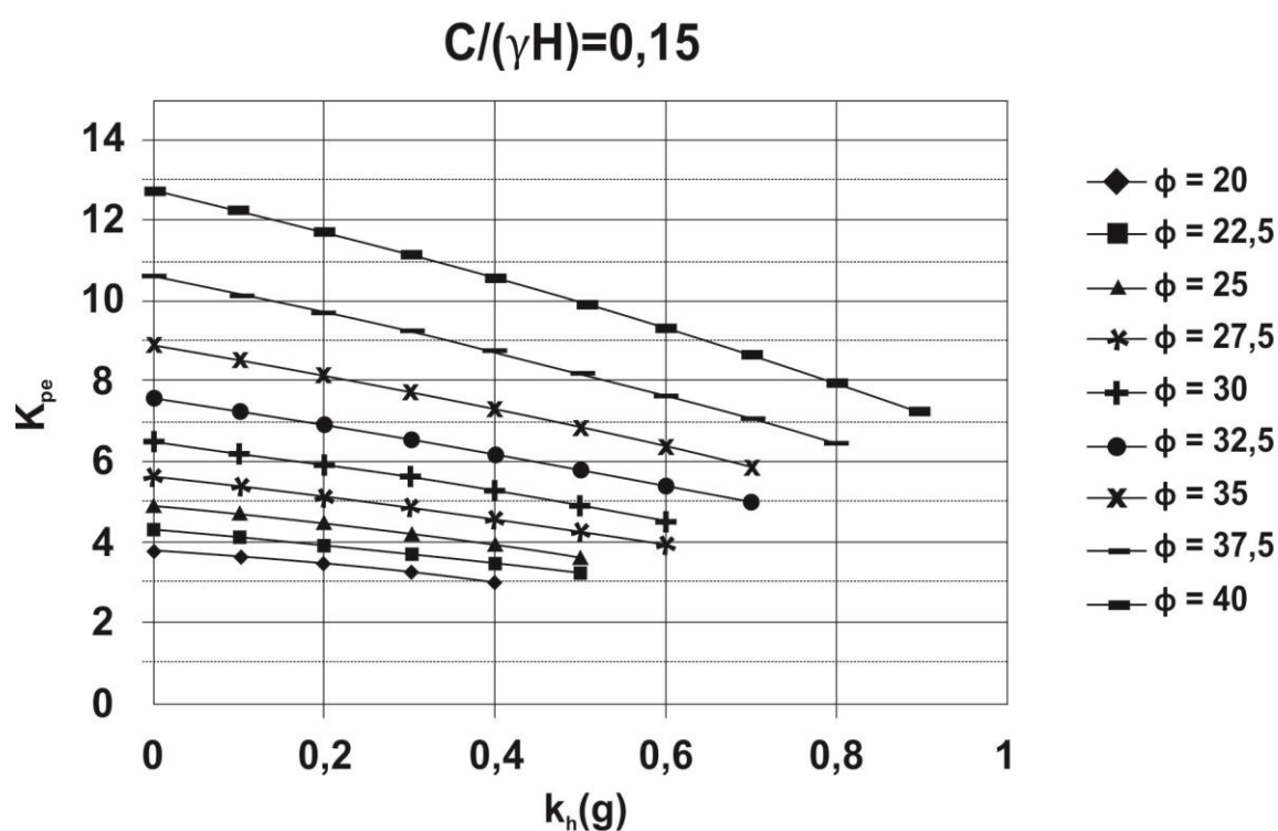
Figura A11.4-3: Coeficiente sísmico de presión pasiva del terreno, basado en el método de la espiral logarítmica, para c/(\gamma H) = 0,10 y 0,15 (c=cohesión del suelo, \gamma =peso unitario del suelo, y H= altura del muro de contención)
