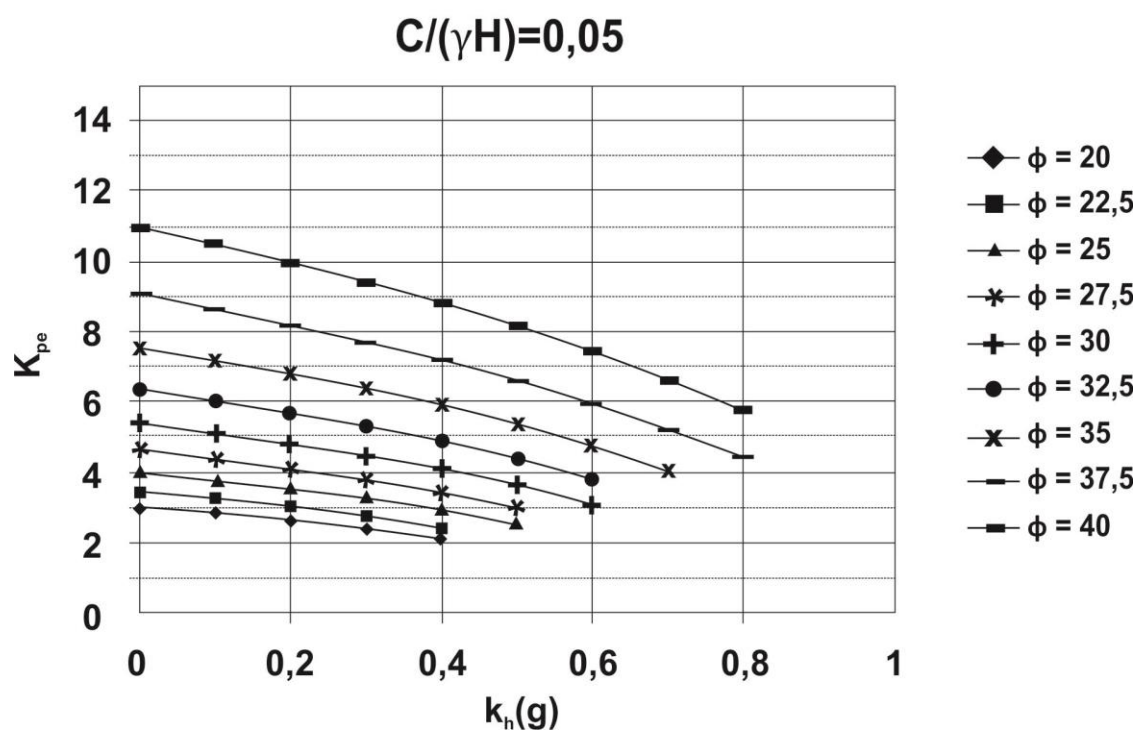
Figura A11.4-2: Coeficiente sísmico de presión pasiva del terreno, basado en el método de la espiral logarítmica, para c/(\gamma H) = 0 y 0,05
