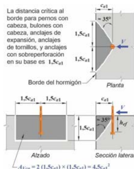
Figura C 17.7.2.1a. Cálculo de A_{Vco} .
