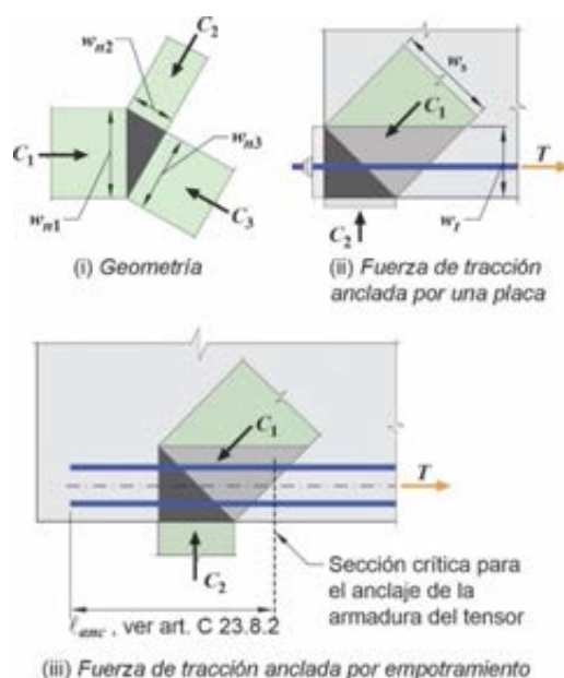
Figura C 23.2.6a. Nodos hidrostáticos. IF-2025-136960277-APN-DNGPO#MOP
