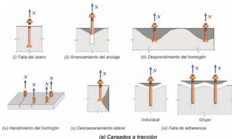
Figura C 17.5.1.2. Modos de falla de anclajes.
