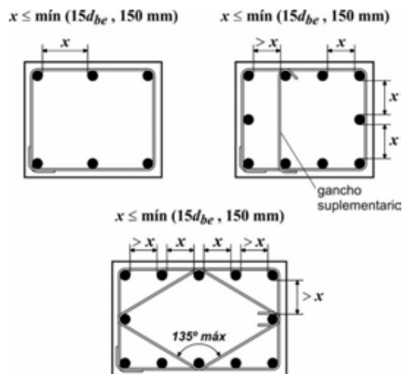
Figura C 25.7.2.3a. Croquis para aclarar las medidas entre barras de columna arriostradas lateralmente y el anclaje de estribos rectilíneos.
