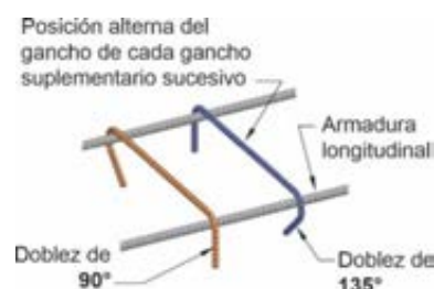
Figura C 25.3.5. Gancho suplementario.
