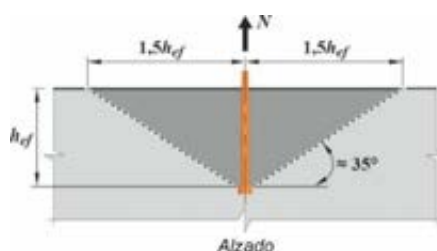
Figura C 17.5.1.3a. Cono de desprendimiento por tracción.
