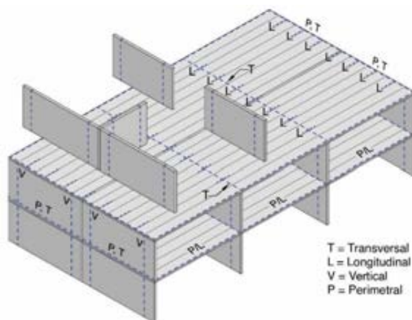
Figura C 16.2.5. Disposición típica de las armaduras de vinculación para integración en estructuras de grandes paneles.
