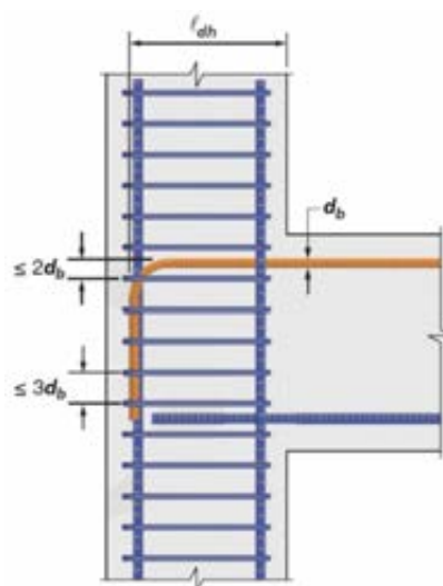
Figura C 25.4.3.2a. Colocación de estribos abiertos o cerrados paralelos a la barra que se desarrolla, separados a lo largo de la longitud de prolongación del gancho más el doblez.
