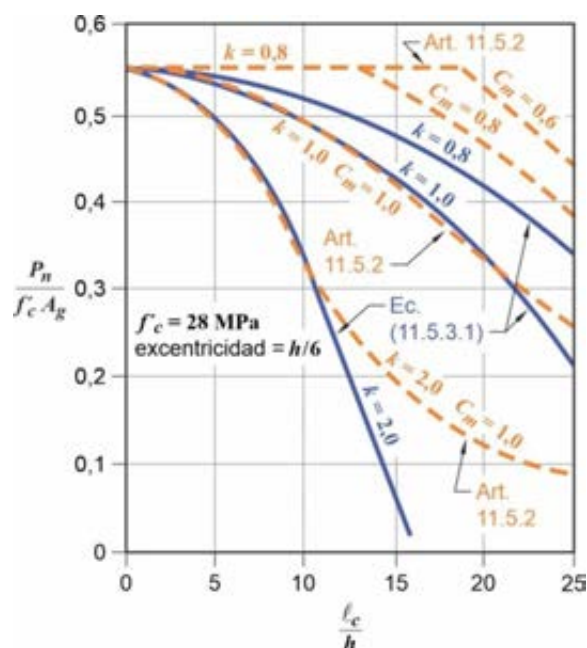
Figura C 11.5.3.1. Diseño simplificado de tabiques, ecuación (11.5.3.1), comparada con el artículo 11.5.2.
