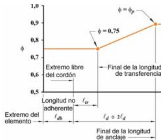
Figura C 21.2.3a. Variación de \phi con la distancia desde el extremo libre del cordón en elementos pretesados con cordones completamente adheridos.
