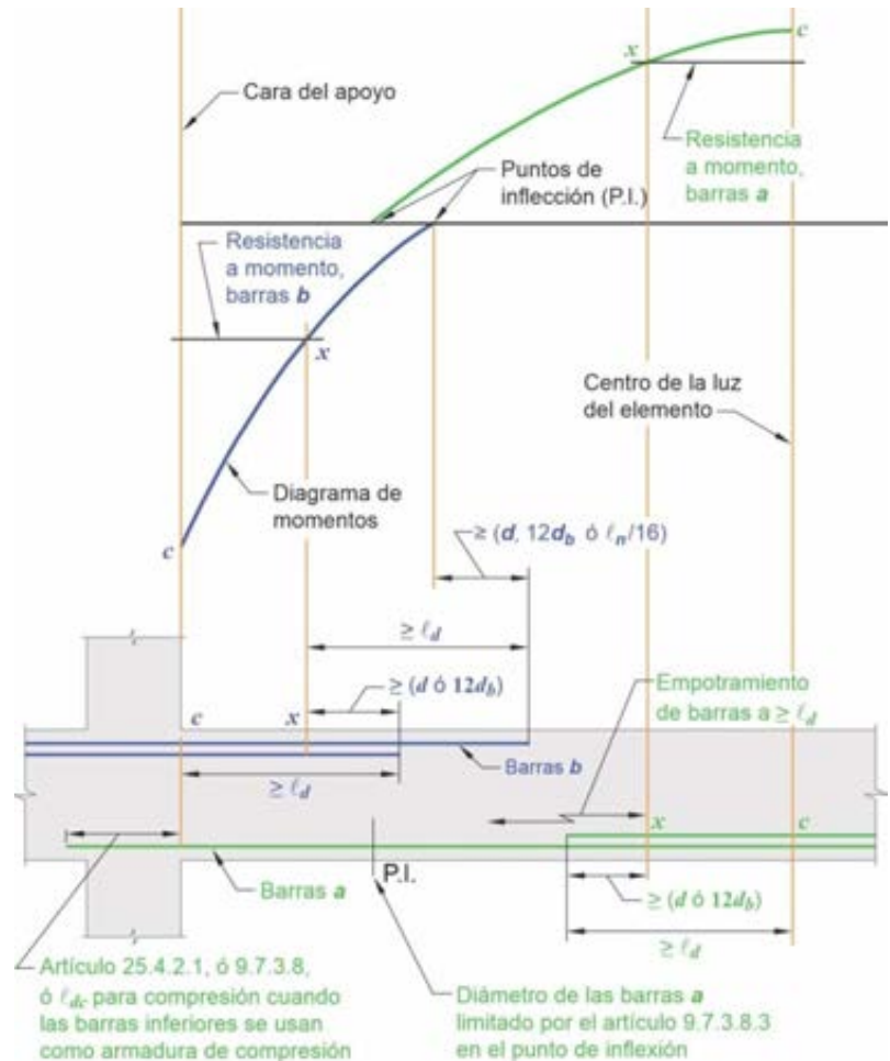
Figura C 9.7.3.2. Longitud de anclaje de la armadura por flexión en una viga continua típica.
