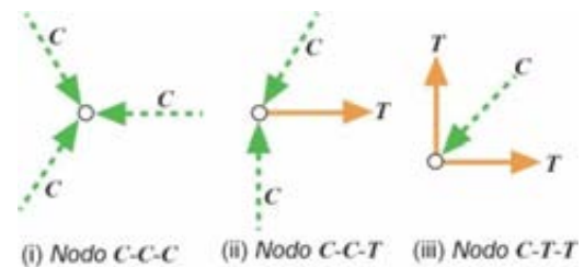
Figura C 23.2.6c. Clasificación de nodos.
