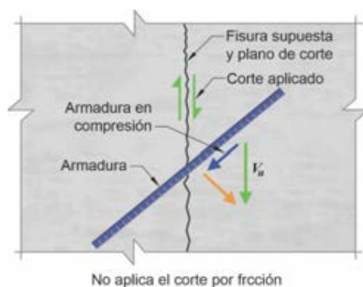
Figura C 22.9.4.3b. Compresión en la armadura de corte por fricción.
