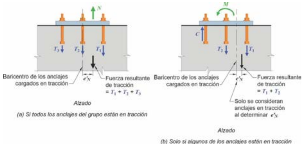
Figura C 17.6.2.3.1. Definición de e'_N para un grupo de anclajes.
