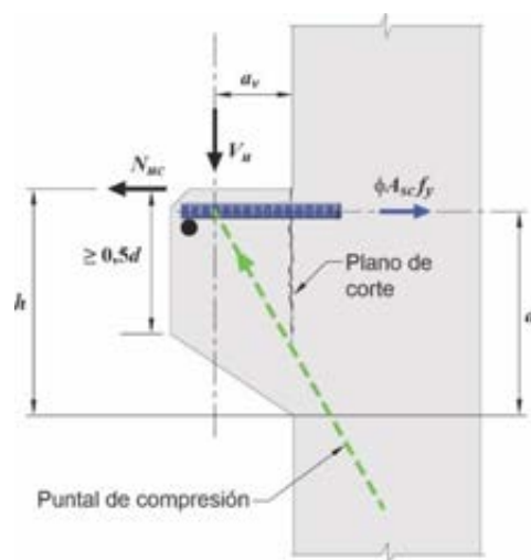
Figura C 16.5.1a. Acción estructural de una ménsula corta.
