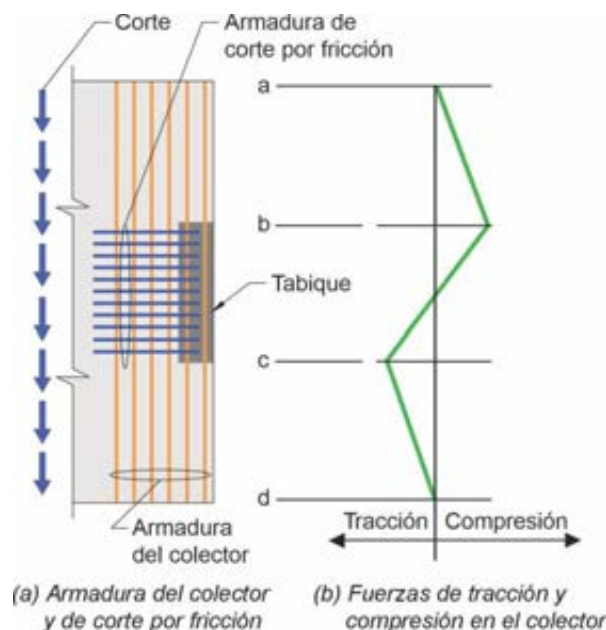
Figura C 12.5.4.1. Colector de altura total y armadura de corte por fricción requerida para transferir las fuerzas del colector al tabique.
