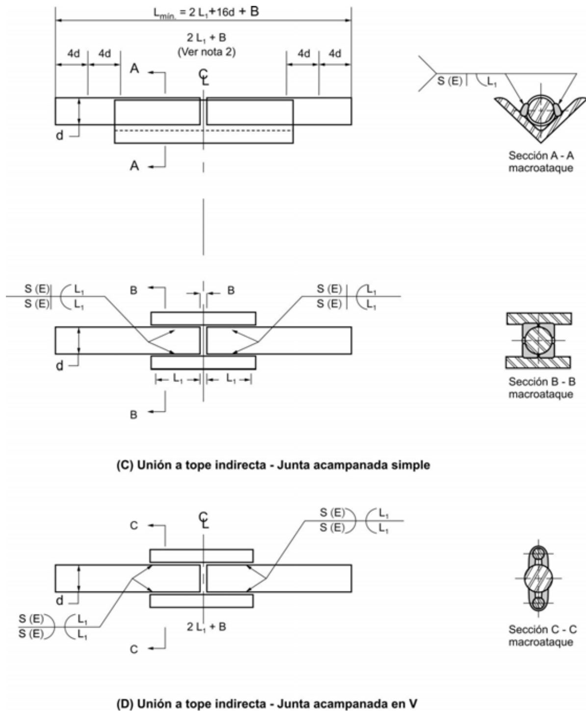
Figura I.4.4. (Continuación). Probetas de soldadura para ensayos de tracción para calificación de EPS.
