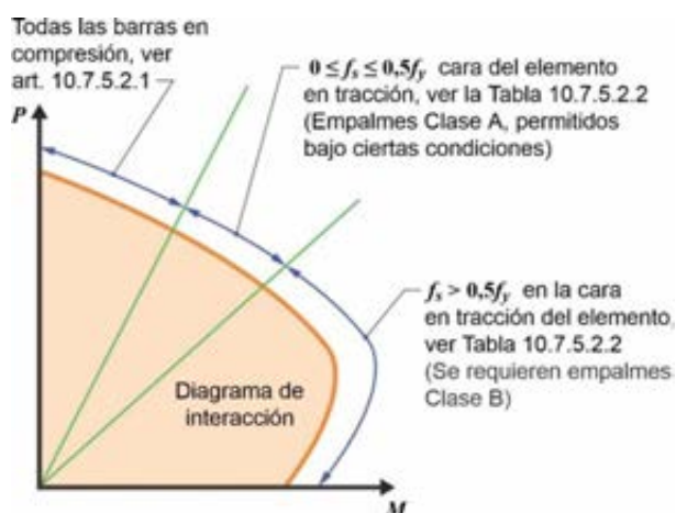
Figura C 10.7.5.2. Requisitos para empalmes por yuxtaposición en columnas.
