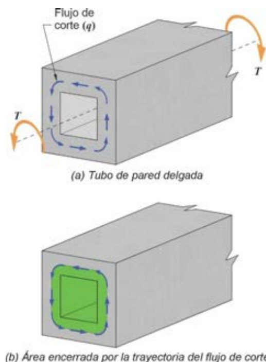
Figura C 22.7. (a) Tubo de pared delgada, y (b) área encerrada por la trayectoria del flujo de corte.
