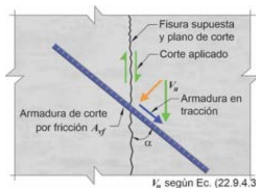
Figura C 22.9.4.3a. Tracción en la armadura de corte por fricción.
