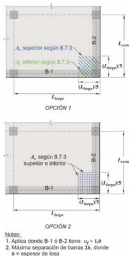
Figura C 8.7.3.1. Armadura de esquina en la losa.
