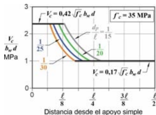
Figura C 22.5.6.2. Aplicación de la Tabla 22.5.6.2 a elementos pretensados cargados uniformemente y con f'_c igual a 35 MPa .
