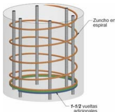
Figura C 25.7.3.4. Anclaje del zuncho en espiral.
