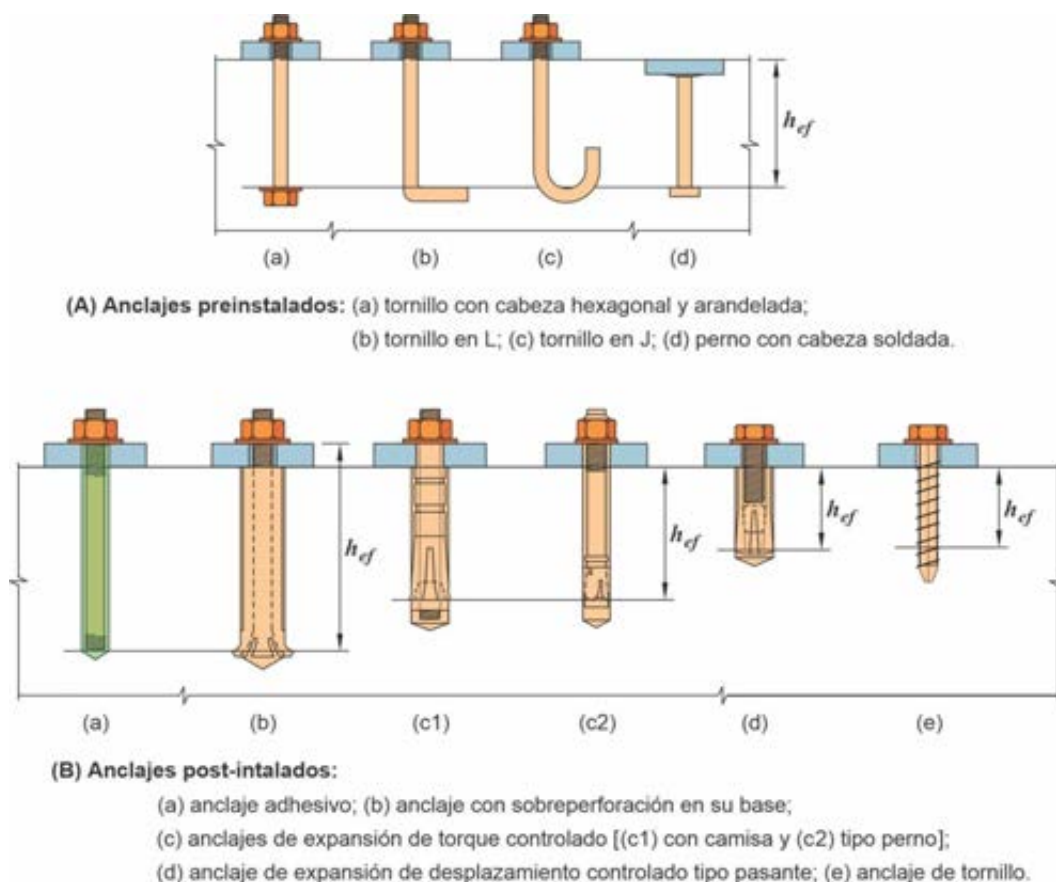
Figura C 2.1. Tipos de anclajes.
