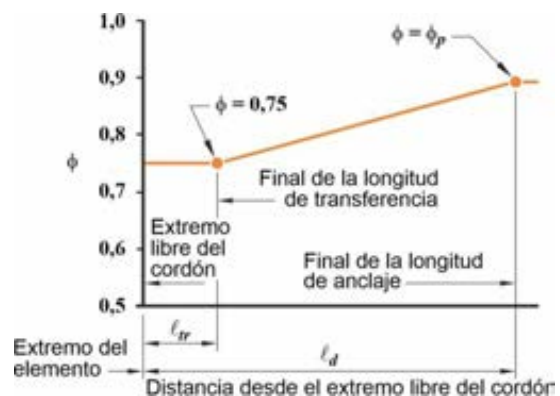
Figura C 21.2.3a. Variación de \phi con la distancia desde el extremo libre del cordón en elementos pretesados con cordones completamente adheridos.
