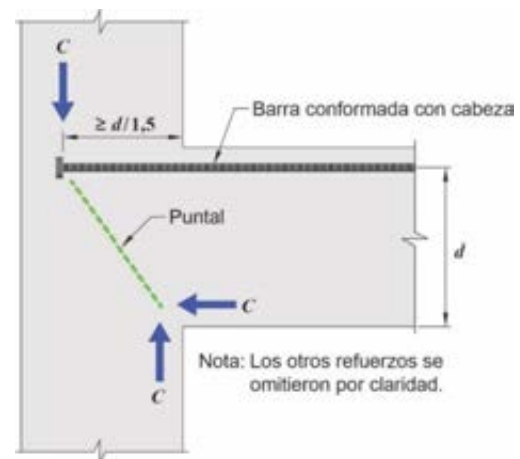
Figura C 25.4.4.2c. Se evita la falla por desprendimiento del hormigón en el nudo, manteniendo una longitud de anclaje mayor o igual a d/1,5 .
