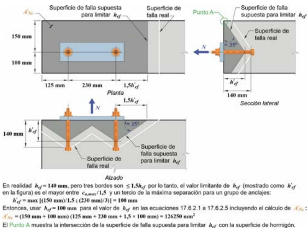
Figura C 17.6.2.1.2. Ejemplo de tracción donde los anclajes están colocados en elementos angostos.
