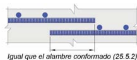
Empalme por yuxtaposición que satisface C 25.5.3.1.1
