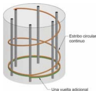
Figura C 25.7.2.3b. Anclaje de estribo continuo.
