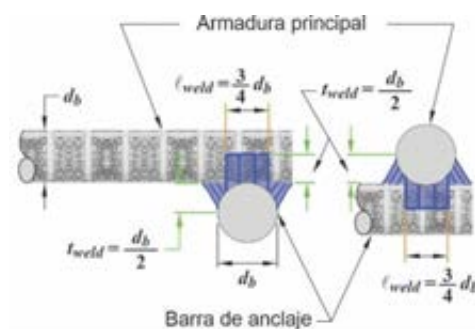
Figura C 16.5.6.3b. Detalles de la soldadura usada en los ensayos de Mattock et al. (1976a).
