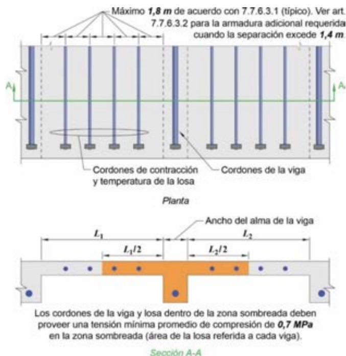
Figura C 7.6.4.2. Sección a través de vigas construidas monolíticamente con la losa.
