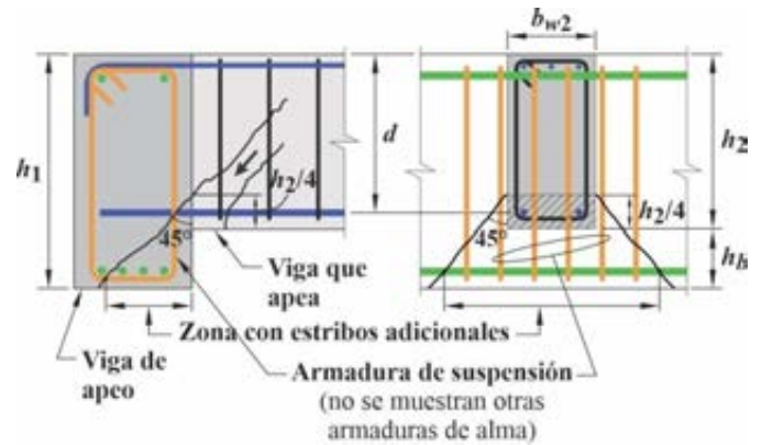
Figura C 9.7.6.2.1. Armadura de suspensión para transferencia de corte.
