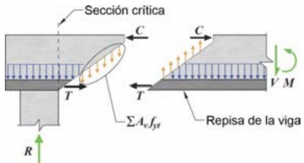
Figura C 9.4.3.2b. Ubicación de la sección crítica de corte en una viga cargada cerca de su cara inferior.
