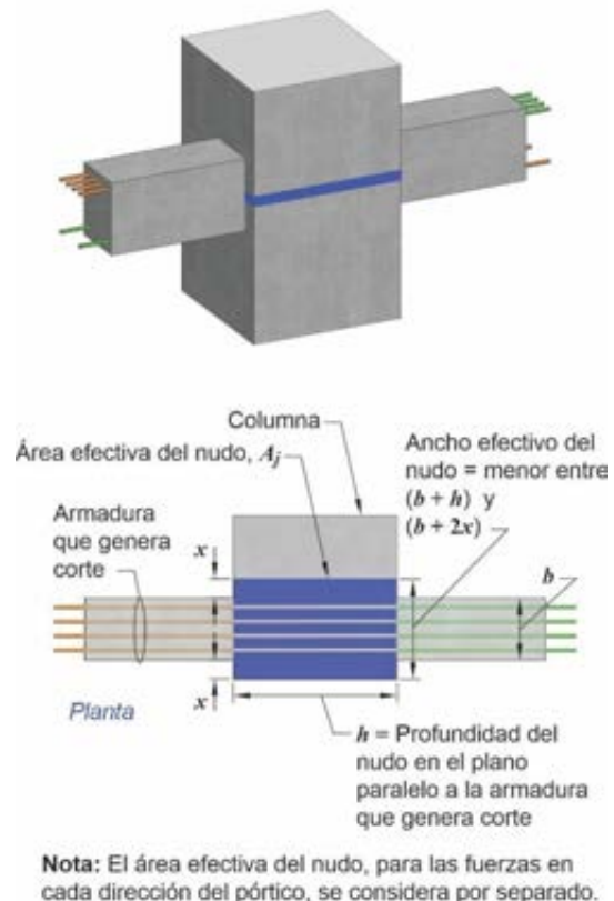
Figura C 15.4.2. Área efectiva del nudo.
