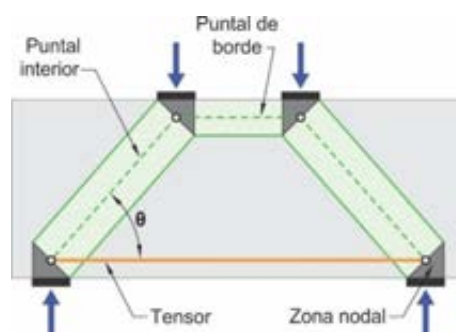
Figura 23.2.1. Descripción del modelo puntal-tensor.
