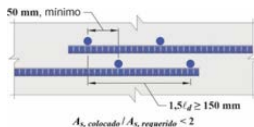
Figura C 25.5.4.1. Empalmes por yuxtaposición de malla de acero soldada de alambres lisos donde: A_{s,colocado} / A_{s,requerido} < 2 .
