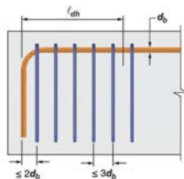
Figura C 25.4.3.2b. Colocación de estribos cerrados o abiertos perpendiculares a la barra que se desarrolla, separados a lo largo de la longitud de desarrollo \ell_{dh} del gancho.
