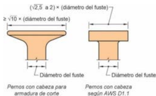
Figura C 20.4.1. Configuraciones de los pernos con cabeza.
