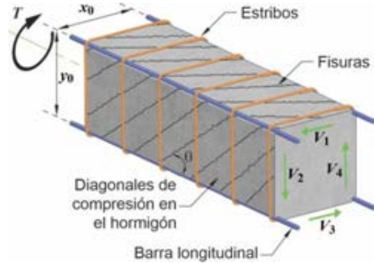
Figura C 22.7.6.1a. Analogía del reticulado espacial.
