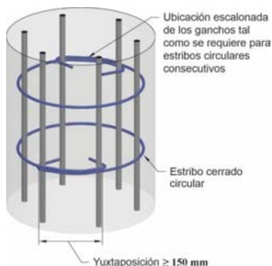
Figura C 25.7.2.4.1. Anclaje de estribos circulares.
