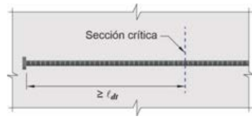
Figura C 25.4.4.2a. Anclaje de barras conformadas con cabeza.
