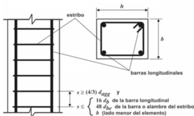
Figura C 25.7.2.1. Separación vertical de los estribos cerrados.
