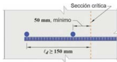
Figura C 25.4.7.2. Longitud de anclaje de la malla de acero soldada de alambres lisos.
