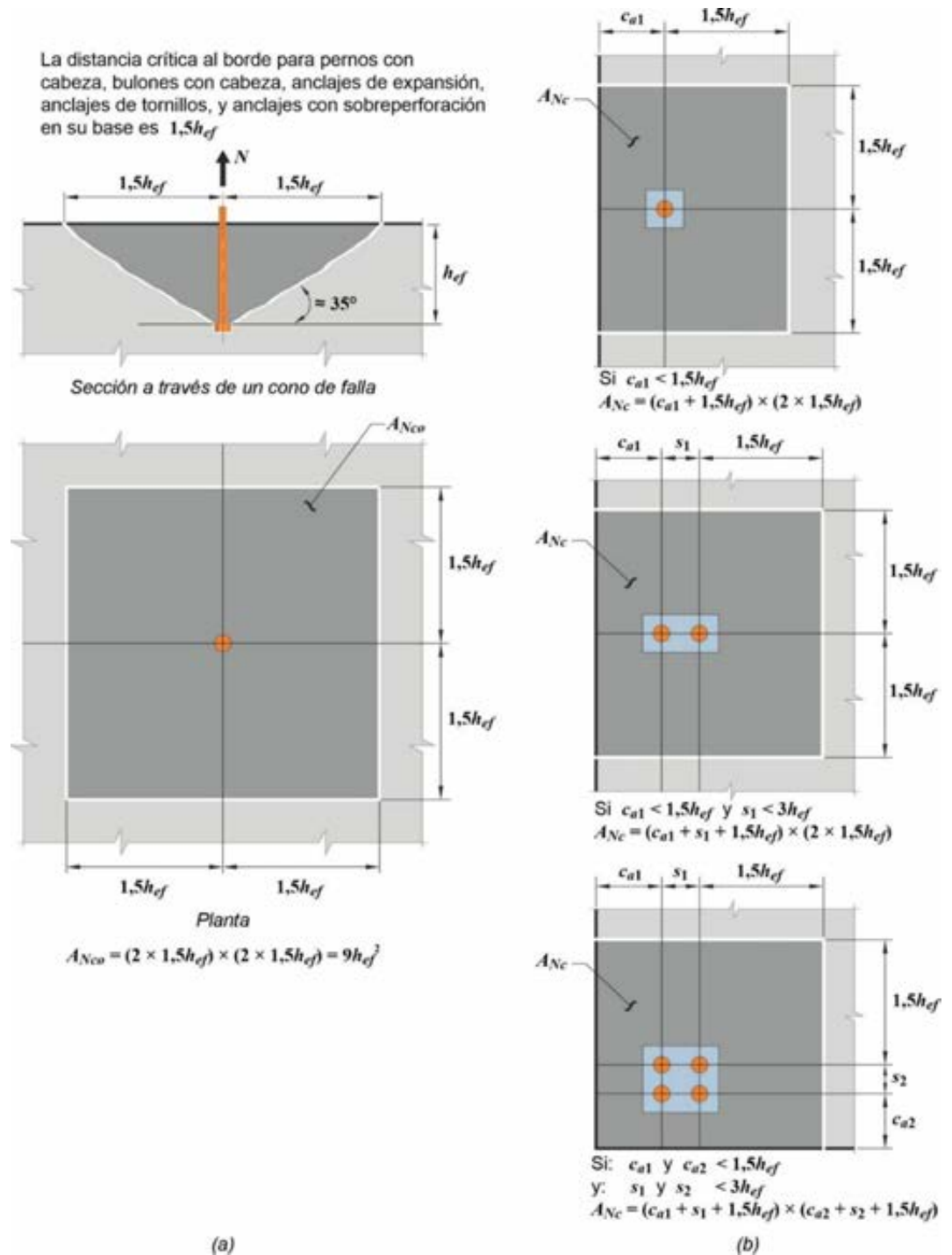
Figura C 17.6.2.1. (a) cálculo de A_{Nco} y (b) cálculo de A_{Nc} para anclajes individuales y grupos de anclajes.
