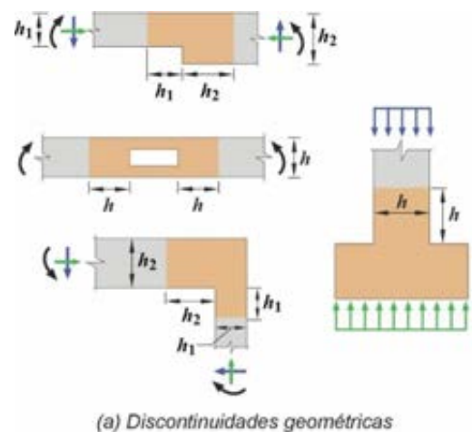
Figura C 23.1(a). Regiones-D y discontinuidades.
