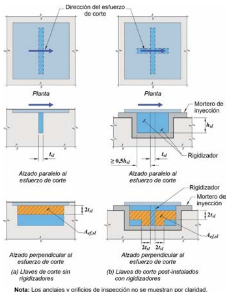
Figura C 17.11.2.1.1. Ejemplos de áreas efectivas de aplastamiento para dispositivos con llaves de corte.
