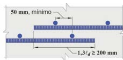
Empalme por yuxtaposición que satisface C 25.5.3.1a
