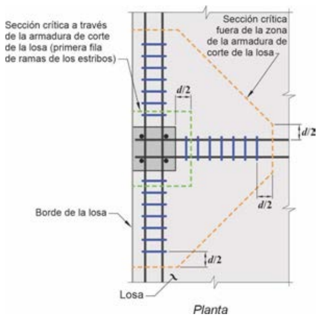
Figura C 22.6.4.2b. Secciones críticas para corte en dos direcciones en losas con armadura de corte en columnas de borde.
