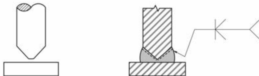
(C) Unión en T - Junta de penetración completa (JPC)
