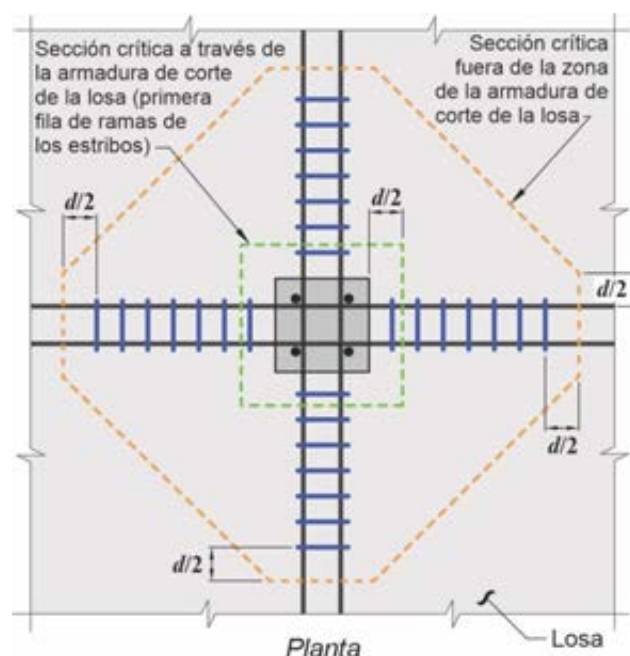
Figura C 22.6.4.2a. Secciones críticas para corte en dos direcciones en losas con armadura de corte en columnas interiores.
