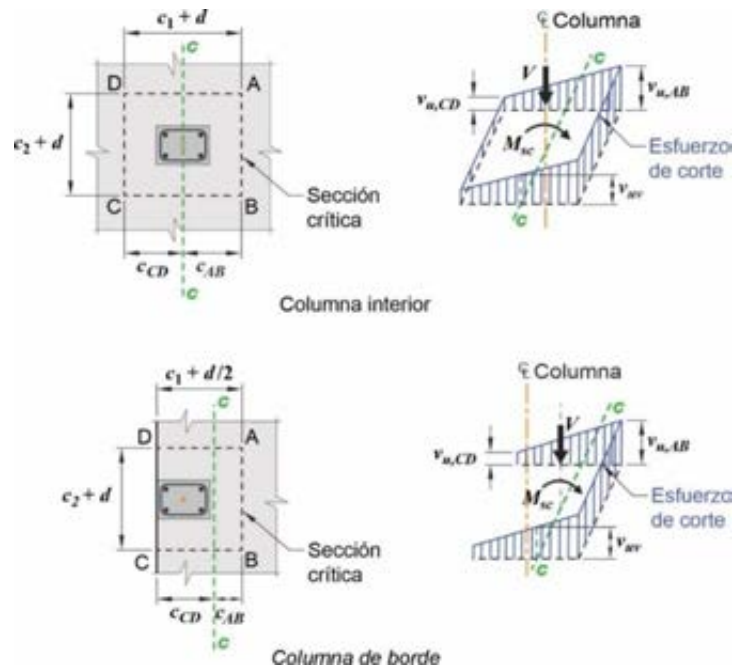
Figura C 8.4.4.2.3. Distribución supuesta de las tensiones de corte.
