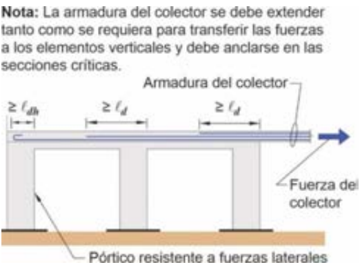
Figura C 12.5.4.3. Esquema de la transferencia de fuerzas del colector hacia los elementos verticales del sistema de resistencia ante fuerzas laterales.
