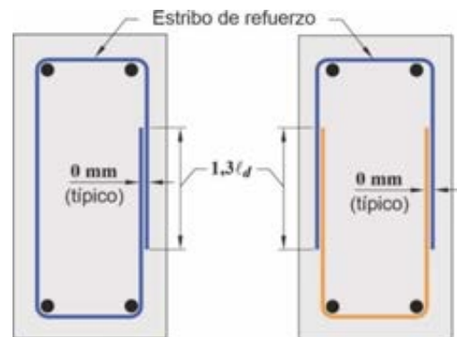
Figura C 25.7.1.7. Configuraciones de estribos cerrados.
