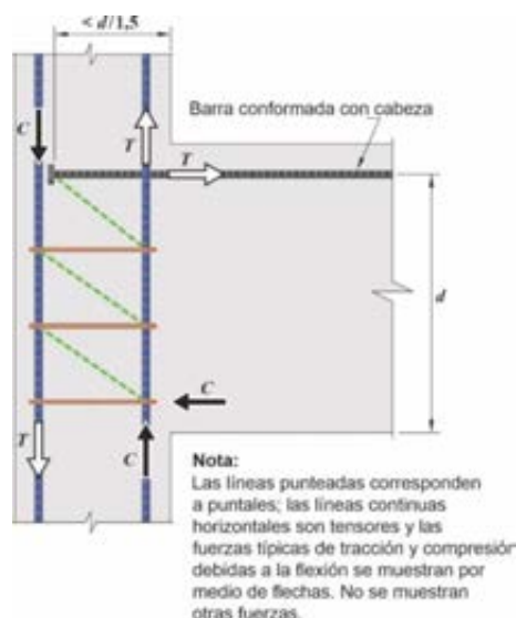
Figura C 25.4.4.2d. Se evita la falla por desprendimiento del hormigón en el nudo, utilizando armadura transversal que habilita un mecanismo puntal-tensor.
