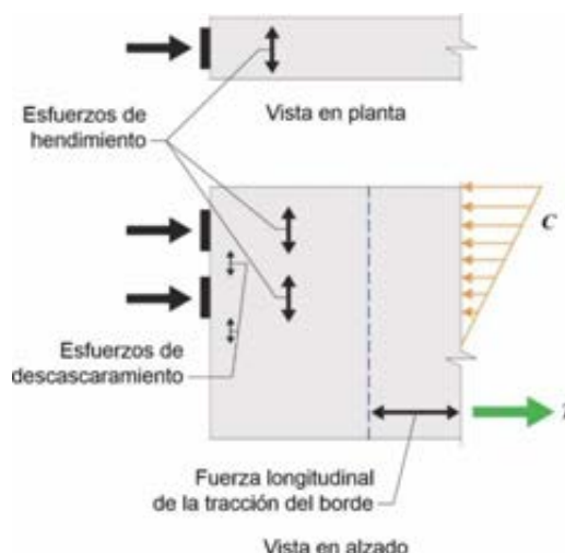
Figura C 25.9.4. Regiones de tensiones de tracción dentro de la zona general.
