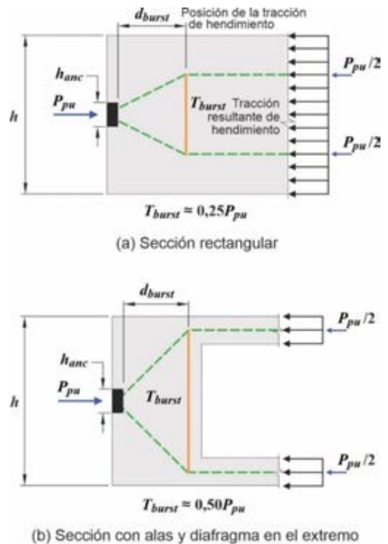
Figura C 25.9.4.4.2. Efecto de los cambios de la sección transversal.
