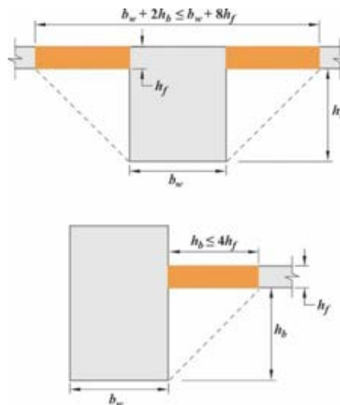
Figura C 8.4.1.8. Ejemplos de la parte de losa que debe incluirse con la viga, según el artículo 8.4.1.8.
