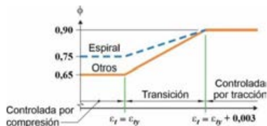
Figura C 21.2.2b. Variación de \phi con la deformación específica neta de tracción en el acero extremo a tracción \varepsilon_t .
