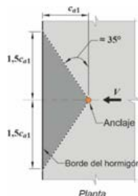
Figura C 17.5.1.3b. Cono de desprendimiento por corte.
