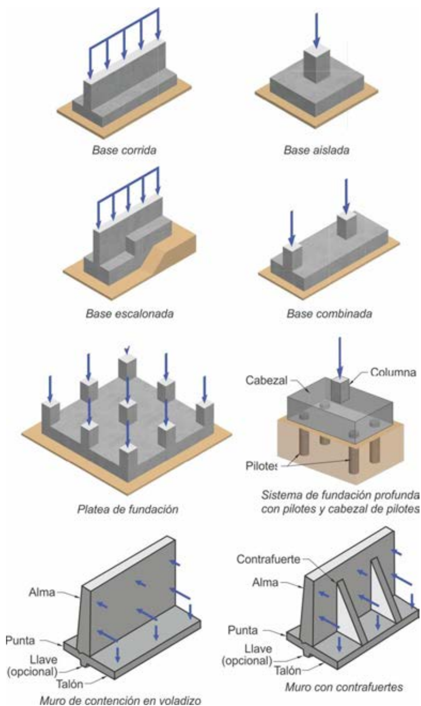
Figura C 13.1.1. Tipos de fundaciones
