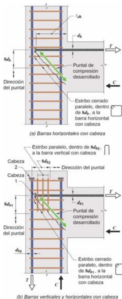
Figura C 25.4.4.4. Estribos abiertos o cerrados colocados paralelos a las barras con cabeza de la viga que se anclan en un nudo viga-columna y que contribuyen a la resistencia de anclaje.
