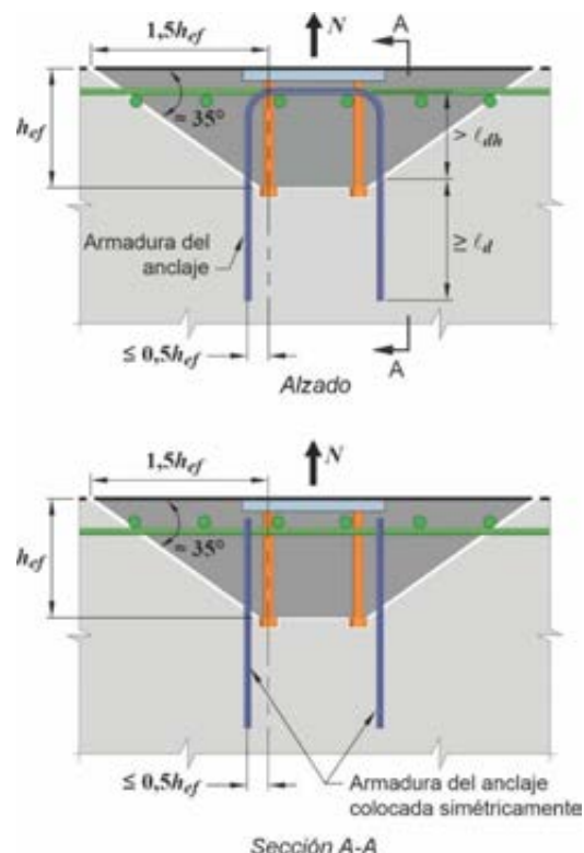
Figura C 17.5.2.1a. Armadura del anclaje para tracción.
