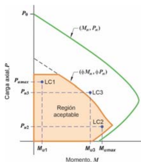
Figura C 10.4.2.1. Combinación de carga crítica en columnas.
