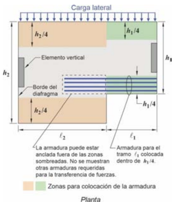
Figura C 12.5.2.3. Ubicaciones de la armadura no pretensada que resiste tracción debida al momento y fuerza axial de acuerdo con el artículo 12.5.2.3.
