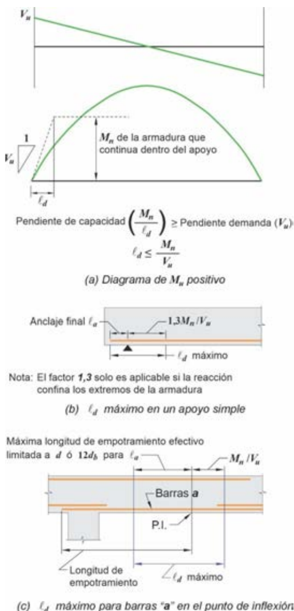
Figura C 9.7.3.8.3. Determinación del diámetro máximo de la barra de acuerdo con el artículo 9.7.3.8.3.
