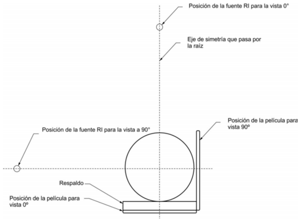
Figura I.5.3. Ubicación de la fuente RI.
