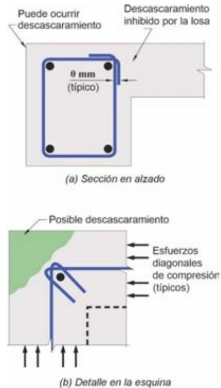
Figura 25.7.1.6. Descascamiento de las esquinas de vigas sometidas a torsión.
