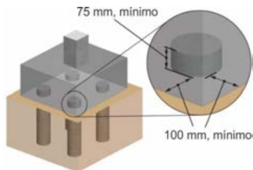
Figura C 13.4.6.3. Empotramiento de los elementos de fundación profunda en el cabezal de pilote.
