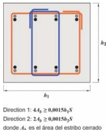
Figura C 10.7.5.2.1. Ejemplo de aplicación del artículo 10.7.5.2.1(a).
