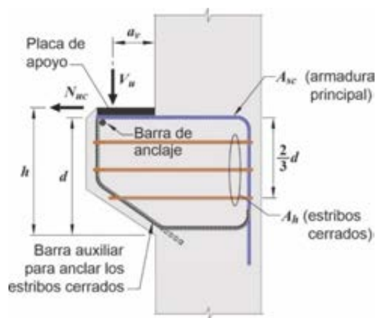
Figura C 16.5.1b. Nomenclatura usada en el artículo 16.5.
