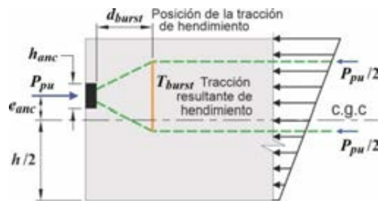
Figura C 25.9.4.3.1. Definición de los términos usados para definir la zona general.
