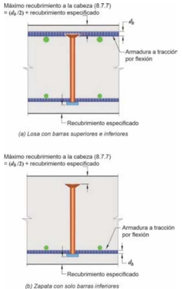
Figura C 20.5.1.3.6. Recubrimiento de hormigón para pernos con cabeza utilizados como armadura de corte.
