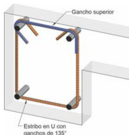
Figura C 9.7.7.1. Ejemplo de estribo de dos piezas que cumple con los requisitos de los artículos 9.7.7.1(c) y 9.7.7.2(b).
