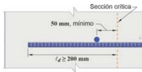
Figura C 25.4.6.3. Anclaje de la malla de acero soldada de alambres conformados.
