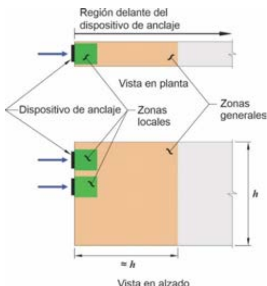
Figura C 25.9.1.1a. Zonas locales y generales.
