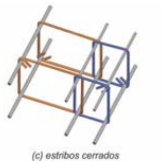
Figura C 8.7.6(c). Estribos cerrados para armadura de corte en losas.
