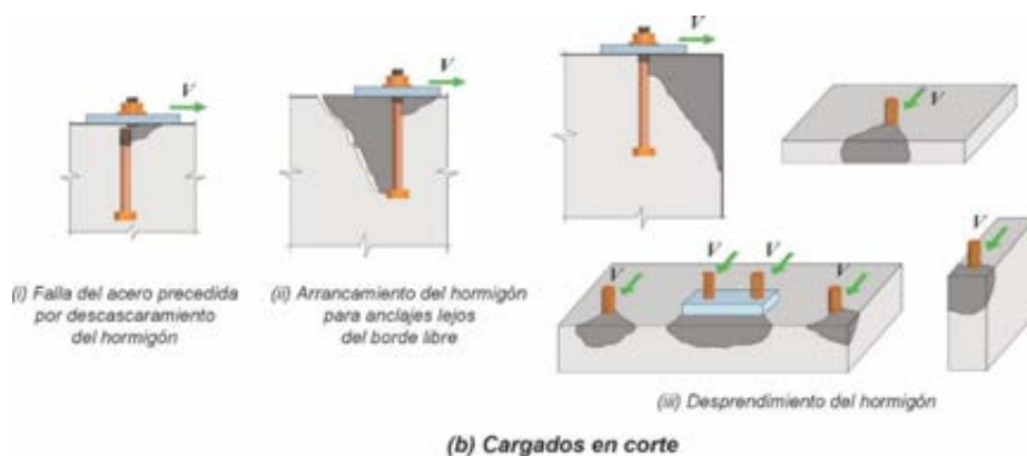
Figura C 17.5.1.2.(Cont.). Modos de falla de anclajes.
