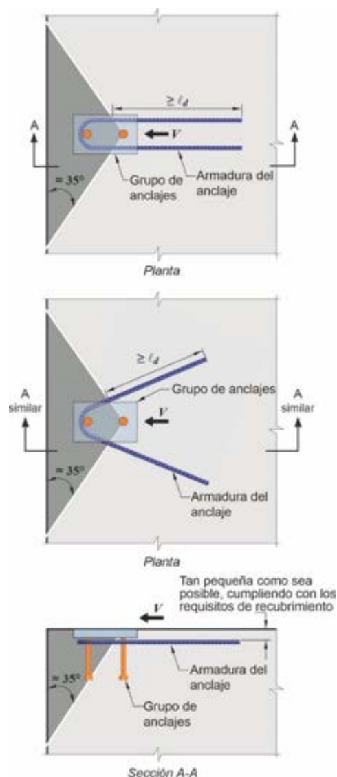
Figura C 17.5.2.1b(i). Armadura del anclaje por corte en forma de horquilla.
