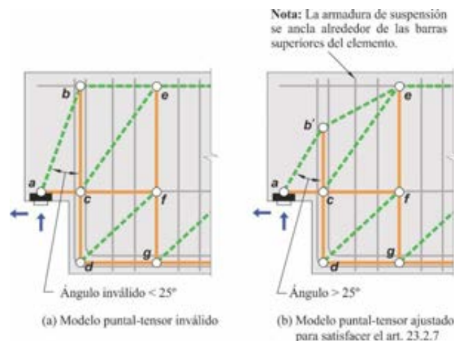
Figura C 23.2.7. Modelo puntal-tensor de una entalladura ilustrando el ajuste requerido para cumplir con el artículo 23.2.7.
