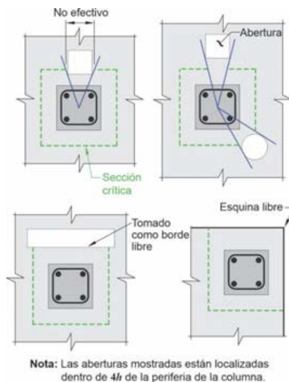
Figura C 22.6.4.3. Efecto de aberturas en la losa y bordes libres (las líneas discontinuas muestran el perímetro efectivo).
