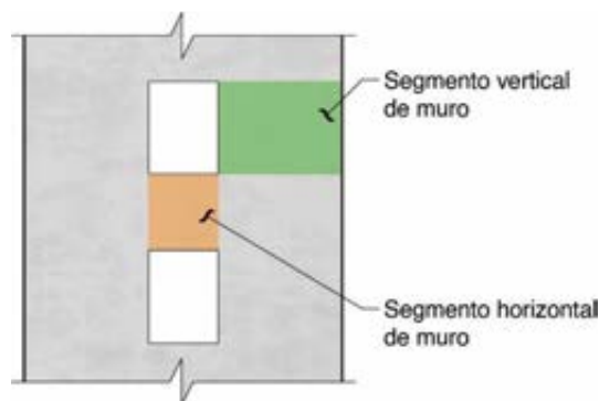
Figura. Muro con aberturas.
