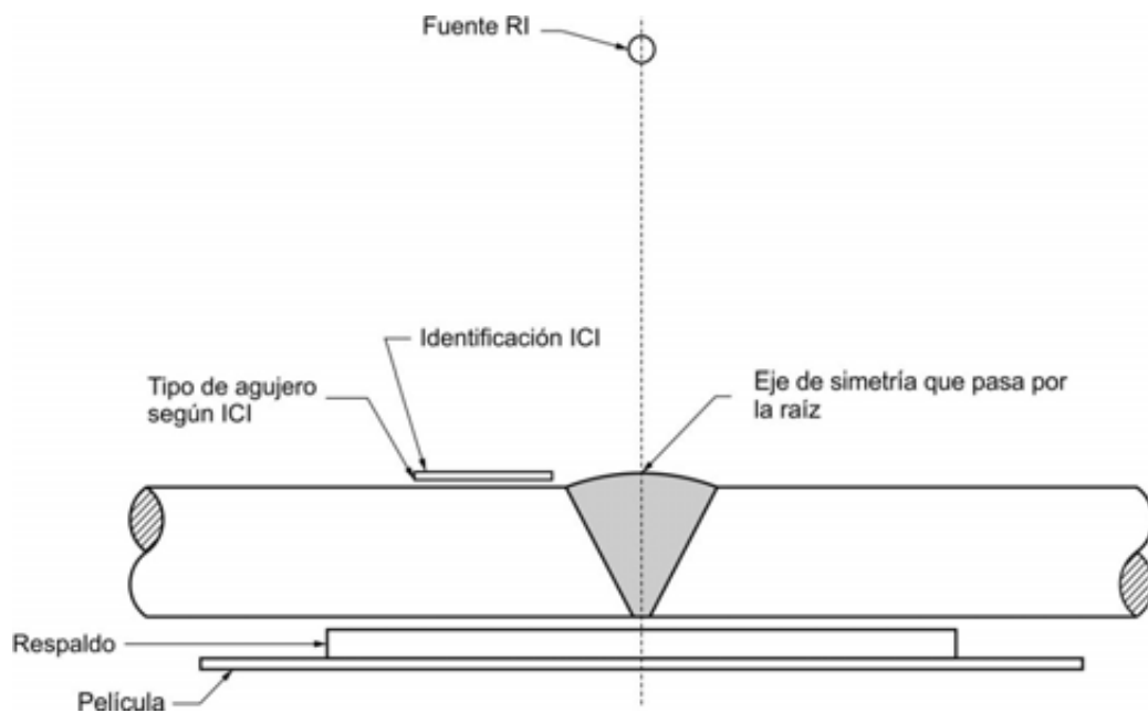
Figura I.5.4. Ubicación de la película.
