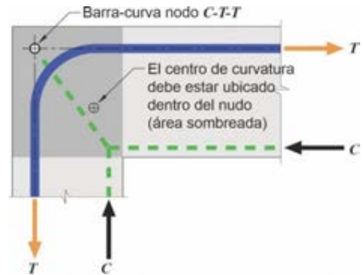
Figura C 23.10.5. Zona donde debe localizarse el centro de curvatura en un nodo de barra curva en la esquina de un pórtico.
